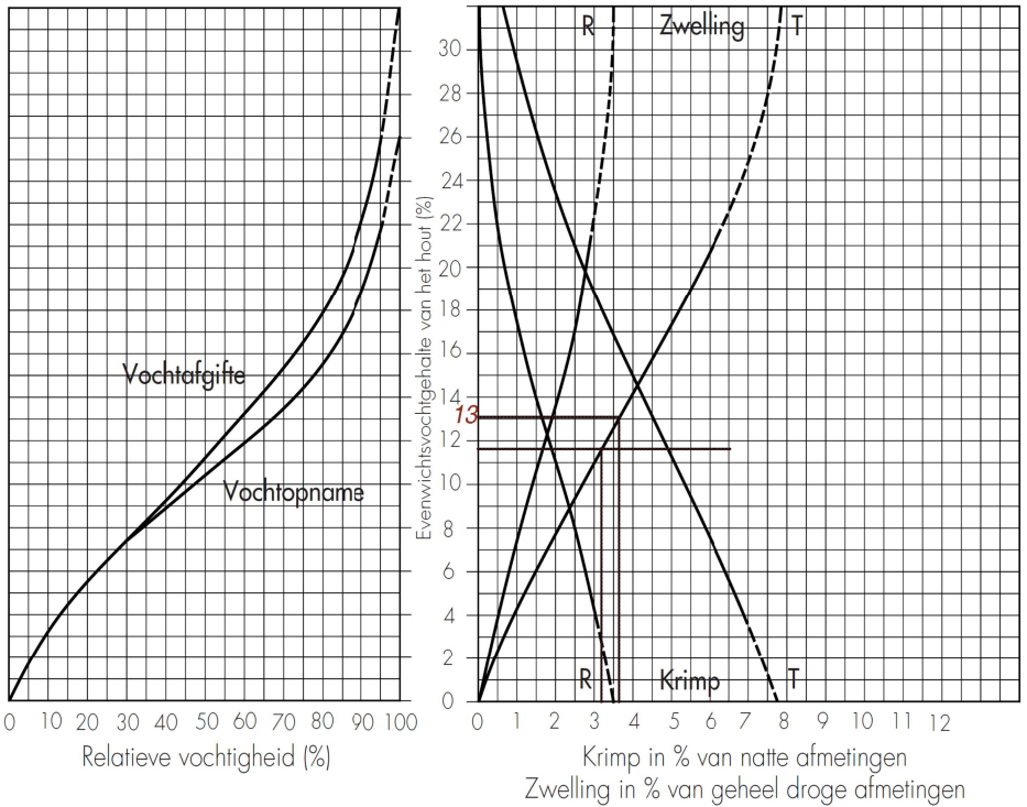
Afb. 24 Relatie tussen het evenwichtsvochtgehalte van het hout en de relatieve luchtvochtigheid [129].
